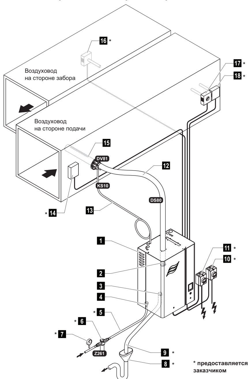
Рис. 2. Система Condaир EL для увлажнения воздуха в воздуховоде
