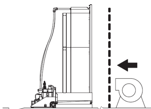
Рис. 16: выбор монтажной позиции относительно вентилятора
