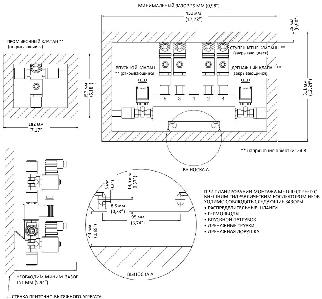
Рис. 13: габариты гидравлического коллектора Condair ME Direct Feed (внешний монтаж) и зазоры
