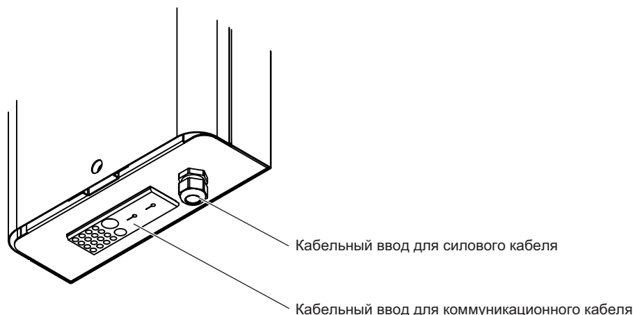
Рис. 20. Ввод кабелей
