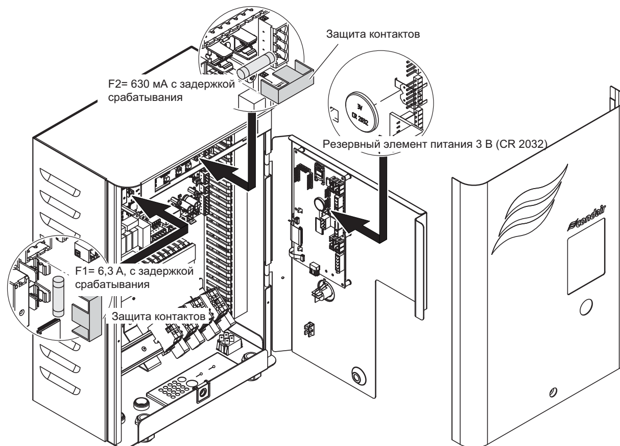
Рис. 10. Замена плавких предохранителей и резервного аккумулятора в блоке управления
