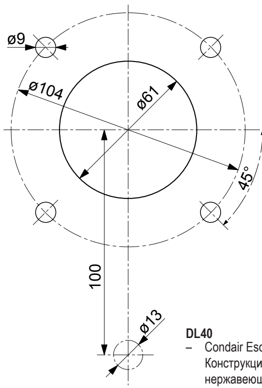
DR73 - Condair Esco 20 Конструкция из нержавеющей стали
