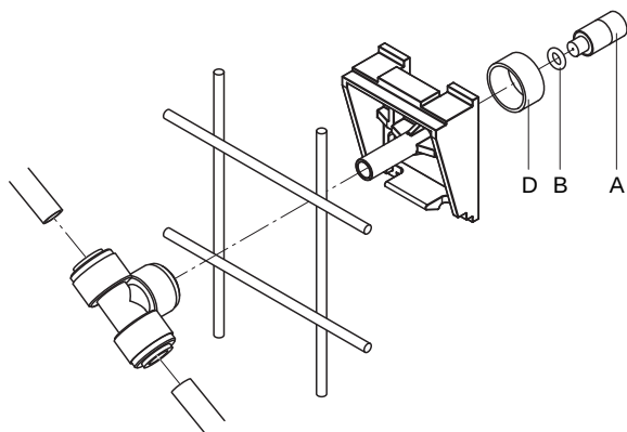
Рис. 14. Демонтаж и монтаж держателя форсунки
