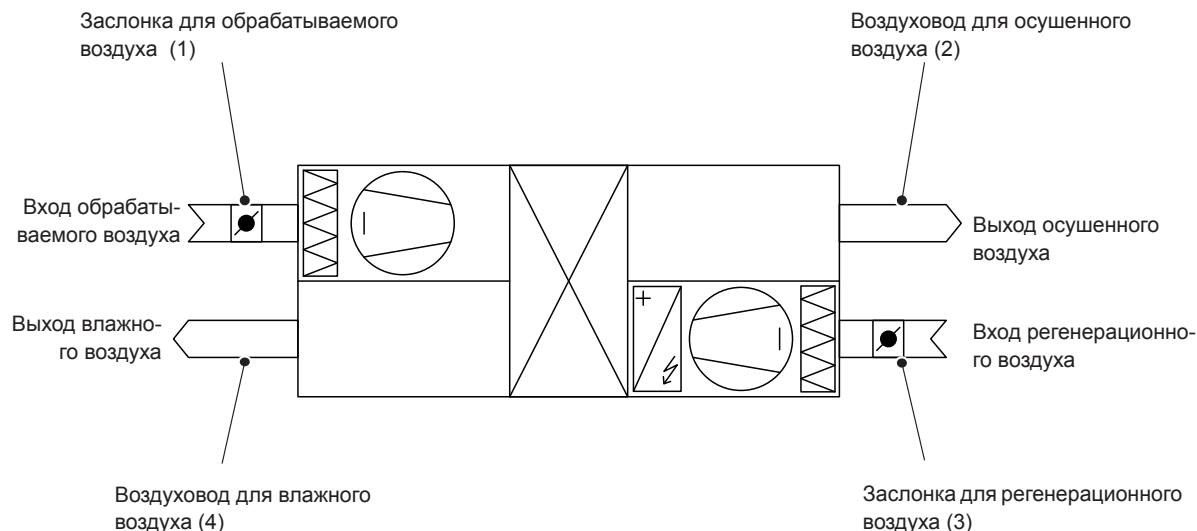
Рис. 3: Схема монтажа
